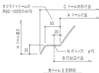
角ドーム E 部詳細
