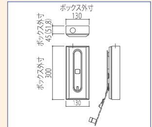
HB-110-R/RD-N 露出ボックスタイプ（オプション）
