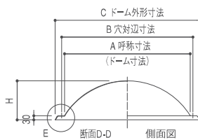
断面D-D 側面図
