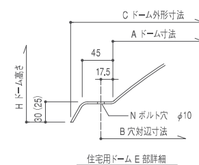
住宅用ドーム E 部詳細
