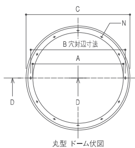
丸型 ドーム伏図
