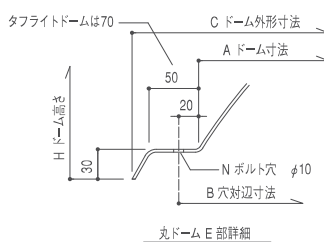
丸ドーム E 部詳細
