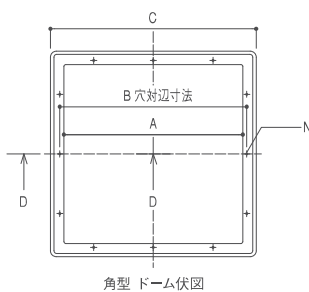
角型 ドーム伏図
