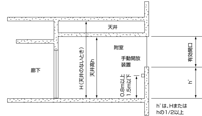
附室排煙窓の設置基準
