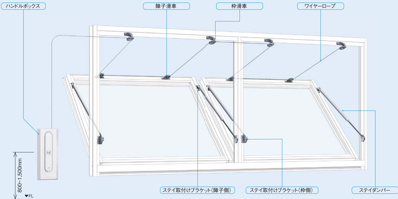
SL80 部品構成表
